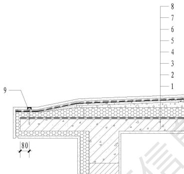
图 B.0.1 檐口
