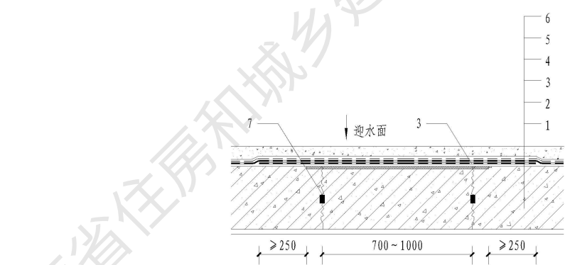
图 D.0.4-2 顶板后浇带
