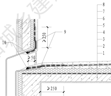
图 B.0.4-1 横式水落口
